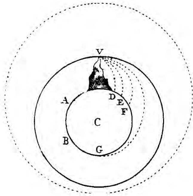
Dessin fait par Newton (Philosophiae Naturalis Principia Mathematica 1687) montrant comment on passe de la chute d'un corps à la satellisation de ce corps
